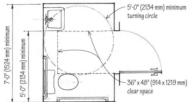
Accessible Toilet Room
