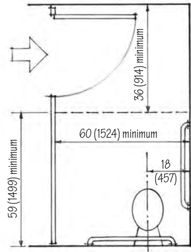
Accessible toilet stall
